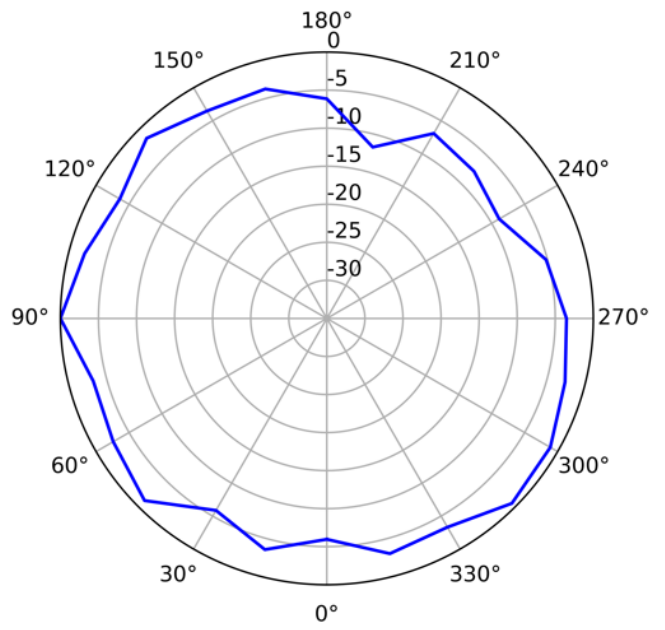
5GHz (Vertical)
